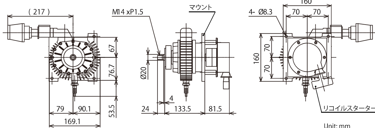
NRG-80 外観寸法図
